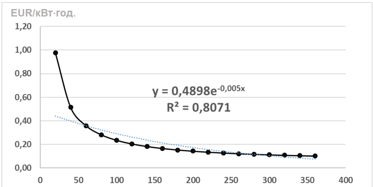
Рис. 3.7. Залежність LCOS від кількості щорічних циклів зарядки-розрядки системи збереження енергії*
